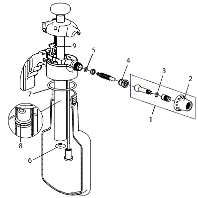
Ring-Set für Super Spray-Matic 1.0 N 12164201
